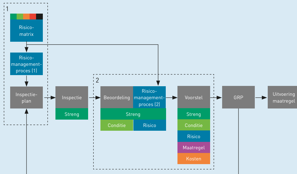
Figuur 2.6 Schema rioleringsbeheer, inclusief risicomanagementtoepassing
