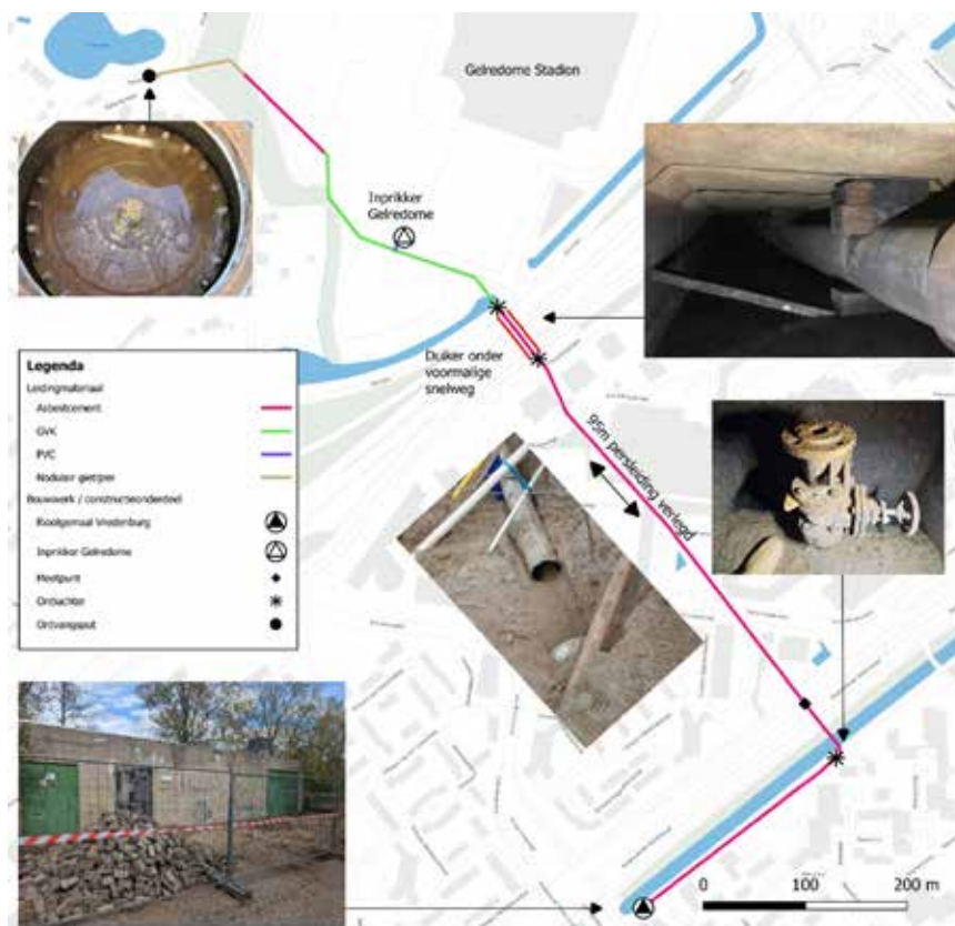
Figuur 5.16 Tracé persleiding Vredenburg. Het tracé begint bij rioolgemaal Vredenburg in het zuiden en eindigt bij de uitstroompuit in het noorden.
