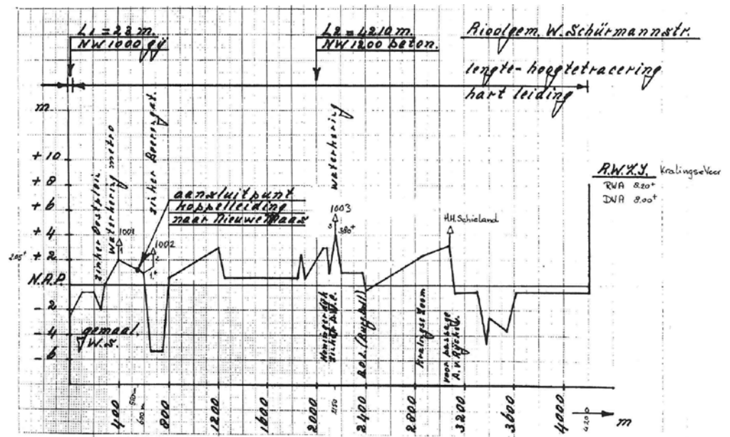
Figuur 4.9 Hoogteligging persleiding Schürmannstraat – rwzi Kralingseveer
