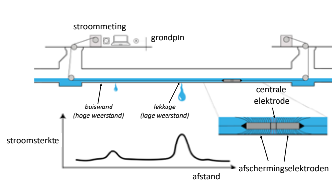
Figuur 5.15 Links: Meetprincipe focused elektrode leak location. Aangepast van Stegeman et al., 2022. Rechts: FELL-meetsonde bij proefopstelling Breda. (Foto: D. Vermeulen, 2022)
