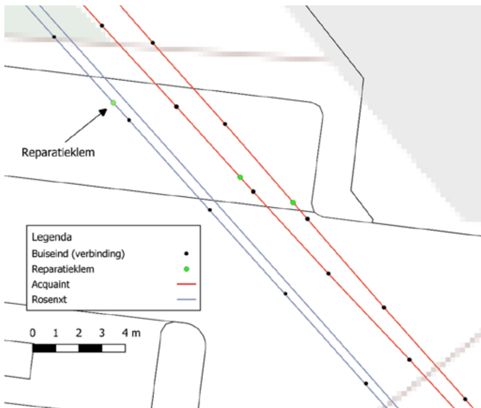
Figuur 5.19 Locatie van dezelfde reparatieklem bij drie verschillende inspecties. De locatie van dit toestandsaspect kan een compleet buisdeel verschoven zijn. Voor Rosenxt is alleen de locatie van verbindingen voor één inspectie ter beschikking gesteld.
