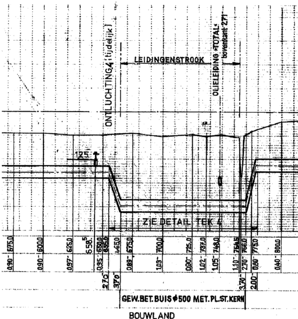
Figuur 3.19 Tekeningen uitvoering leiding bij kruising leidingenstrook, inclusief overgangen wel-niet onderheid
