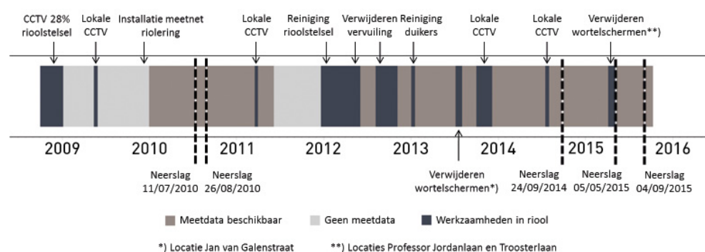
Figuur 3.2 Beschikbaarheid van meetdata, uitgevoerde werkzaamheden en gebruikte neerslaggebeurtenissen meetnet rioolsysteem Tuindorp in de periode 1 oktober 2008 tot en met 6 oktober 2015
